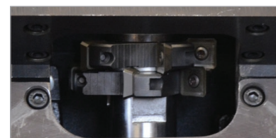
Tête à deux disques de coupe, avec chacun cinq plaquettes de coupe à 4 faces
