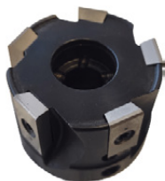
Tête de fraisage équipée de 5 plaquettes de coupe prête à l'emploi
